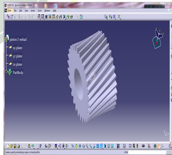
Fig. 6. Pinion 2
